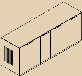
L x W 180x52 H 73 Incluye estantes interiores / Included interiors shelves Madera / Lacado Wood / Lacquered
