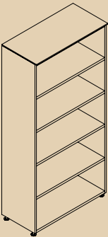
L x W 90x45 H 172 Madera / Lacado Wood / Lacquered
