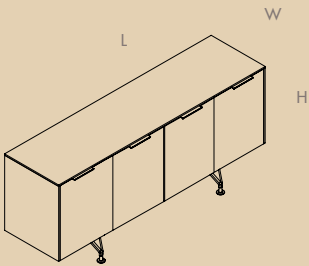
L x W 150x45 / 180x45 H 73 Incluye estantes interiores / Included interiors shelves Madera / Lacado / Pie Metal Wood / Lacquered / Metal Leg
